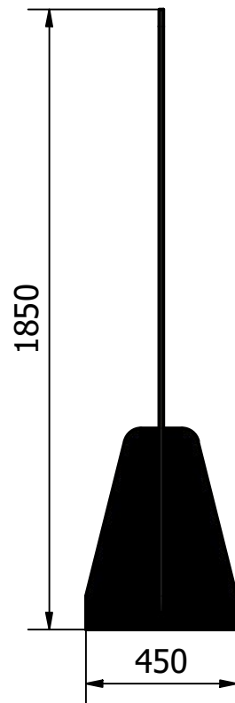
Zijaanzicht
