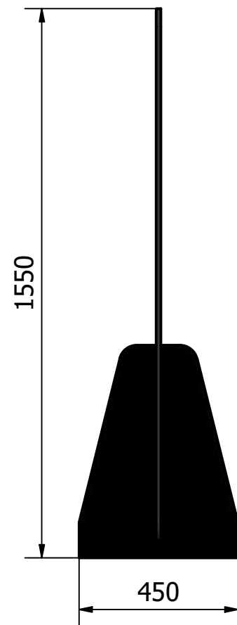
Zijaanzicht
